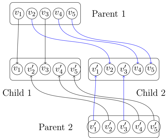
FIGURE 6.4 – Croisement donnant deux enfants
