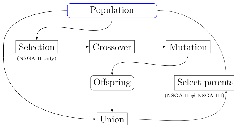
FIGURE 6.1 – Schéma général d'une itération des algorithmes NSGA-II and NSGA-III
