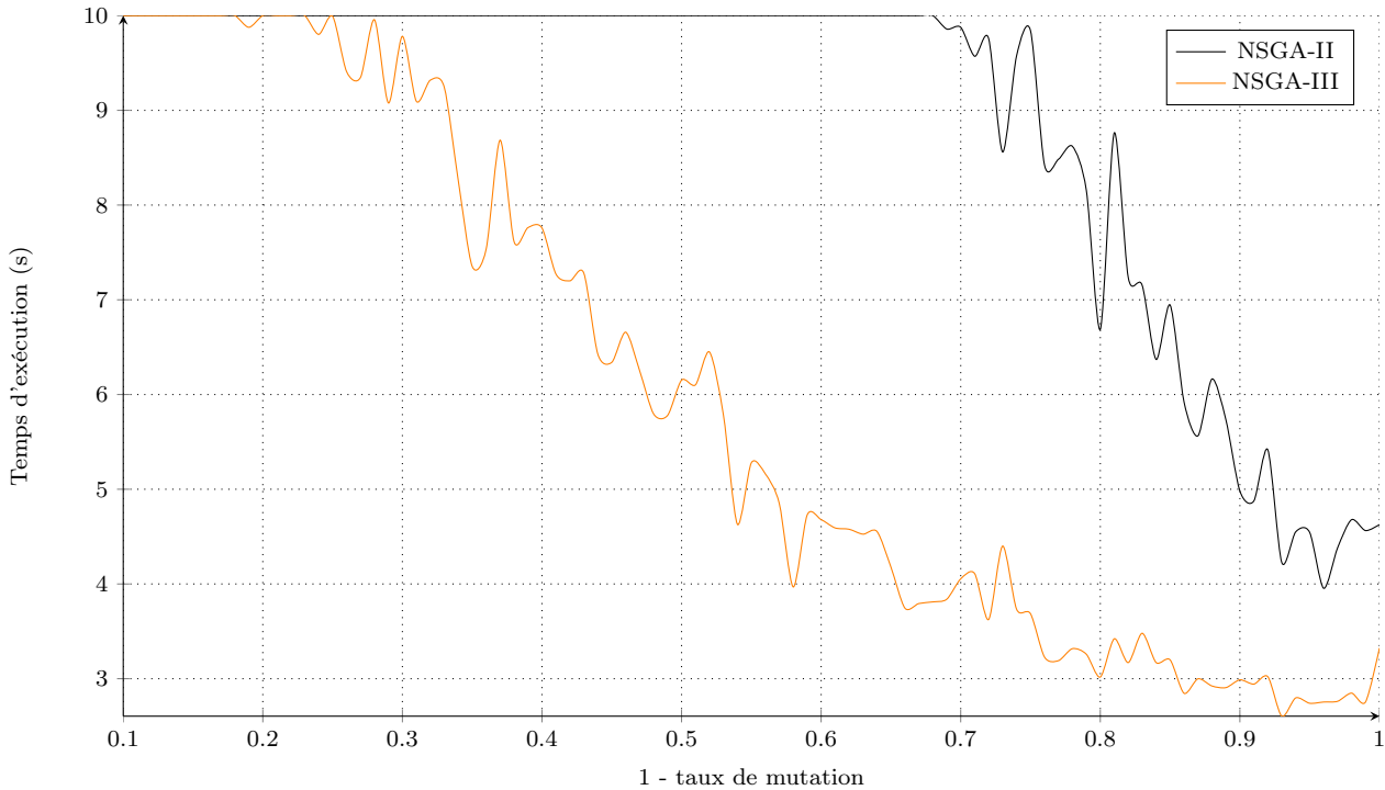
FIGURE 8.3 – Temps d'exécution en fonction de (1 - taux de mutation) (Exemple : Godaddy S_1 )
