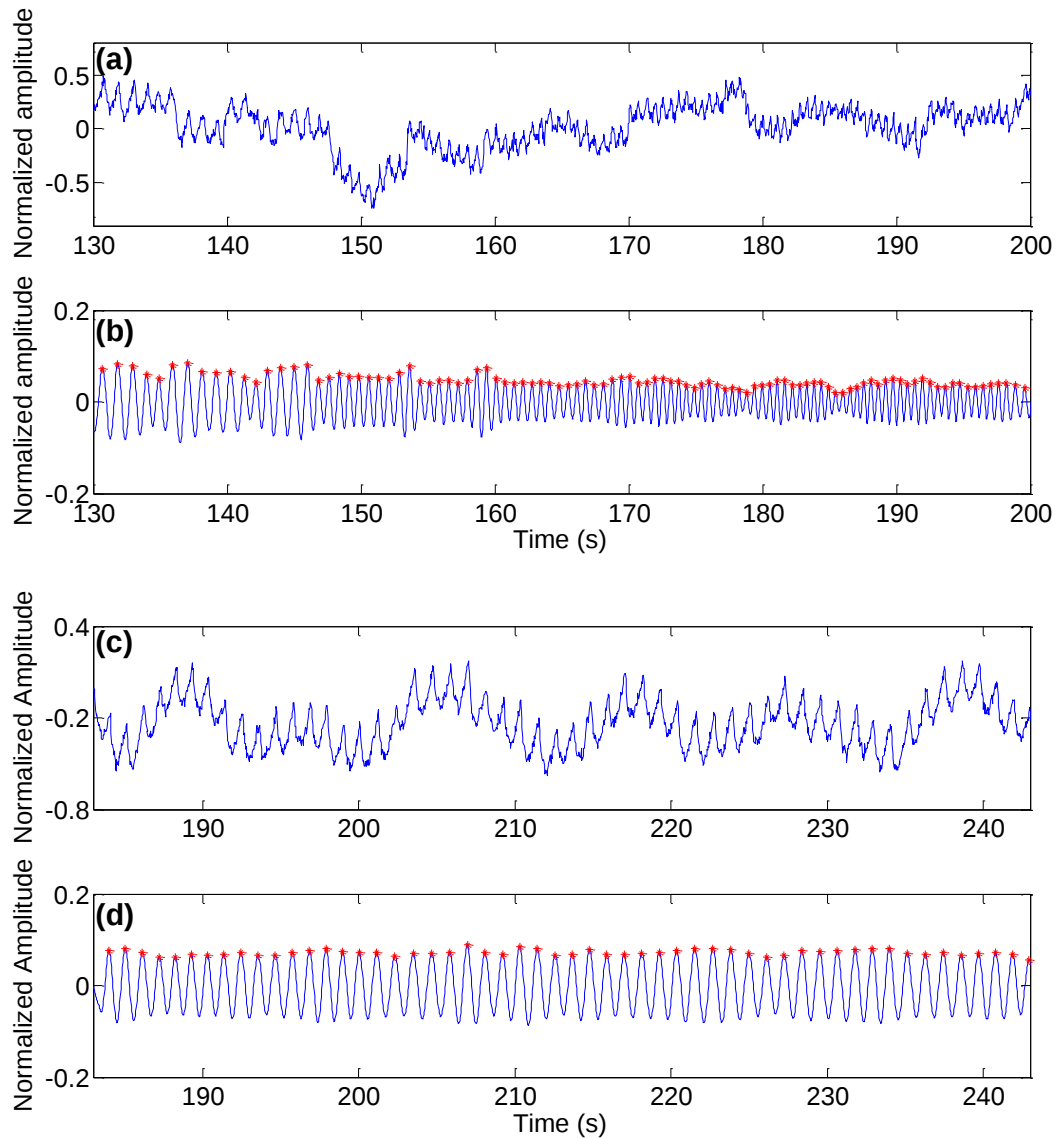
FIGURE 3.29 – Exemple de signaux filtrés. Les signaux bruts peuvent présenter plus (a) ou moins (c) de variations de fréquence et d’amplitude dans le temps. Le filtre permet de supprimer les tendances basses fréquences ainsi que les bruits hautes fréquences [(b) et (d)] tout en conservant les informations importantes.
