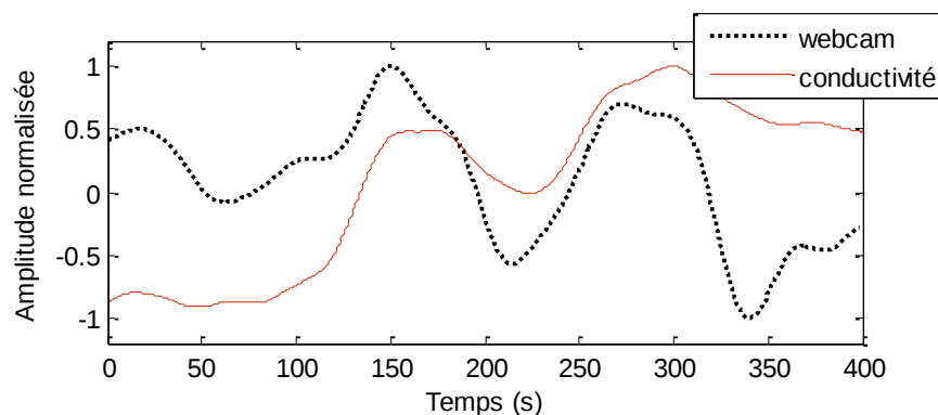
FIGURE 4.12 – Tendance des signaux sur les corrélations. Ces courbes sont tirées du participant n° 7 et ne sont à priori pas corrélées ( r < 0.01 ). Une similitude entre la courbe de stress de chaque capteur est néanmoins clairement identifiable. La mauvaise corrélation est entraînée par la tendance générale des courbes qui pourrait être supprimée pour améliorer ce taux.
