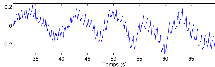
FIGURE 3.22 – Exemple de signal photopléthysmographique extrait d'une webcam. Chaque point de ce signal correspond à la moyenne spatiale d'une trame.
