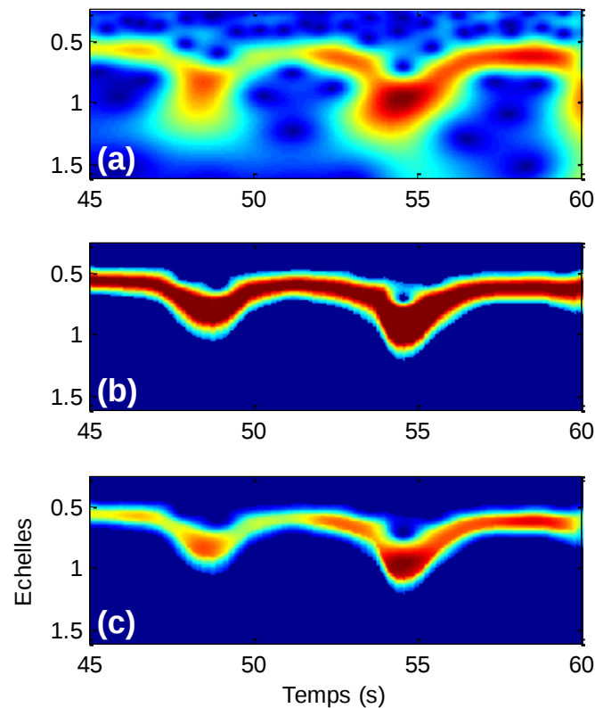
FIGURE 3.28 – Application du filtre sur la transformée en ondelettes d’origine. Le module de la transformée (a) est utilisé pour calculer un filtre en ondelettes (b) permettant de suivre les évolutions de fréquence et d’amplitude du signal photopléthysmographique (c).
